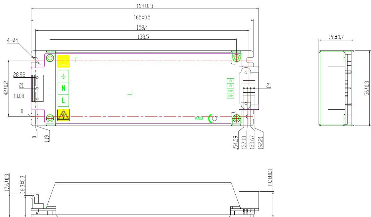
外形尺寸及安装孔——端子坐标图
